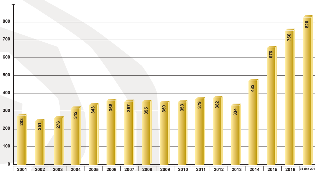
▲ Medlemsutvikling fra 2001-2016
